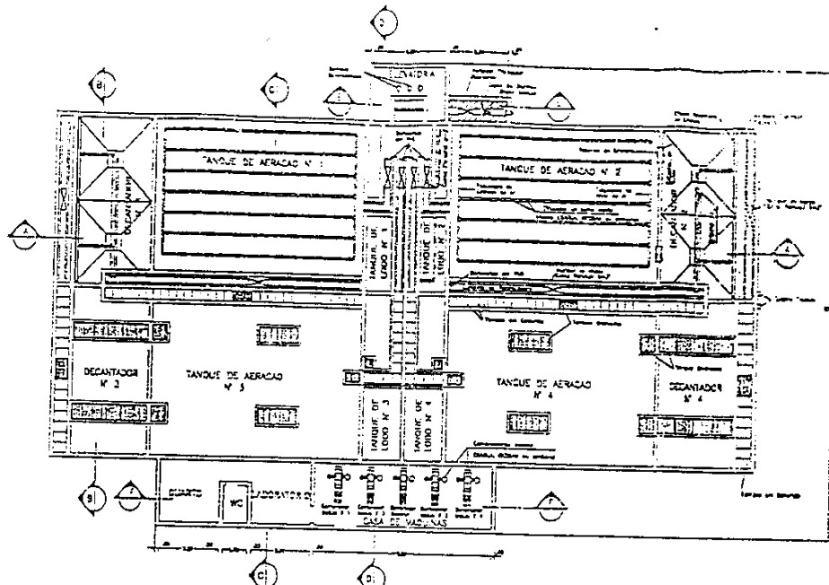
PLANTA BAIXA E TAMPOAMENTO
