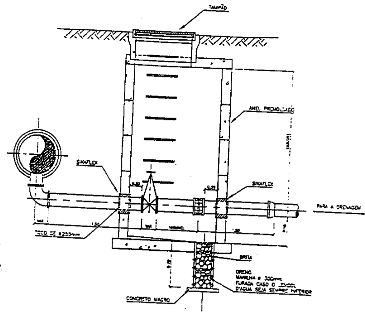
CORTE BB S/ESCALA
