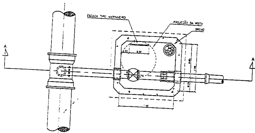
PLANTA S/ESCALA
