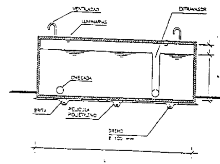
CORTE AA
