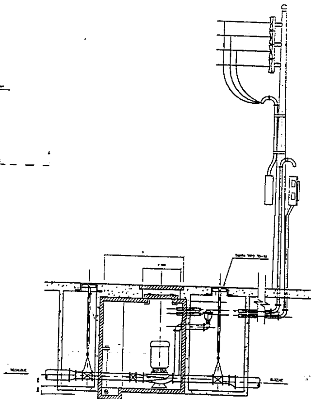
CORTE A-A
