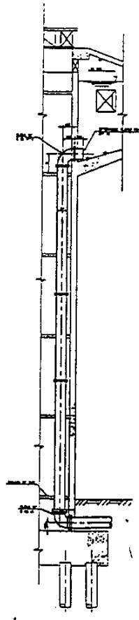
CORTE B-B
