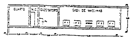
CORTE - FF
